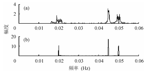
图 4 信号的边际谱
