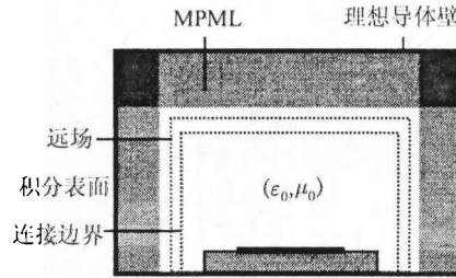
图4 微带天线的 FDTD 计算域设置
