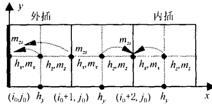
图1 Yee 氏网格中的内插和外插表
