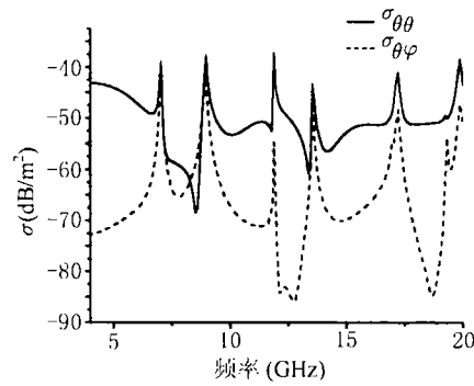
图7 宽基板微带天线的 RCS
