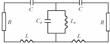
图 5 半波长矩形同轴腔的等效电路
