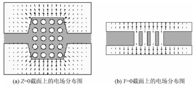
图 4 半波长矩形同轴腔模型的电场分布
