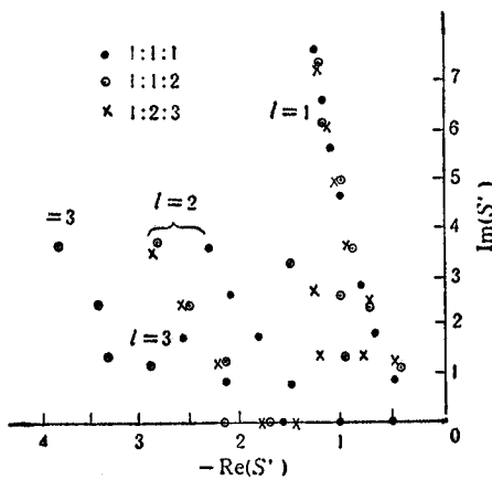
图 2 导体椭球的自然频率 ( l 为层数; S' = S_c/\nu )
